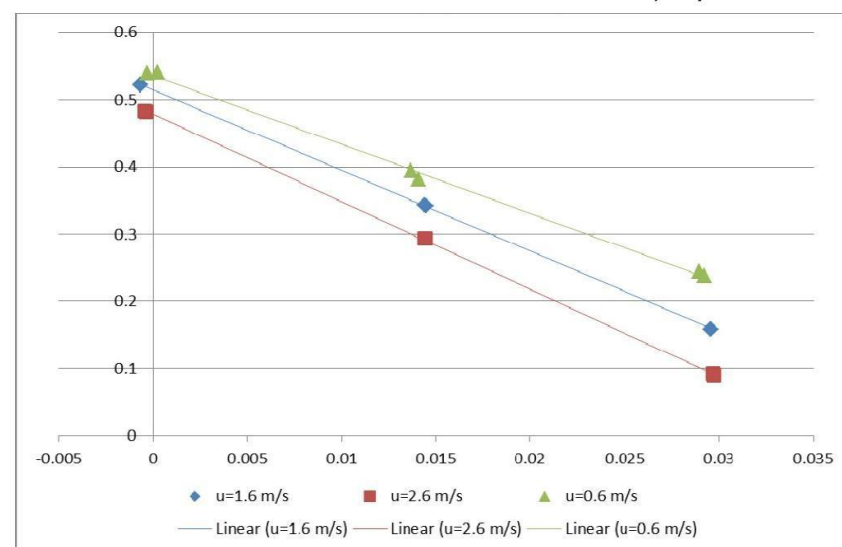
POMIAR PUNKTU WYDAJNOŚCI PRZY G = 884,9\text{W}/\text{m}^2
