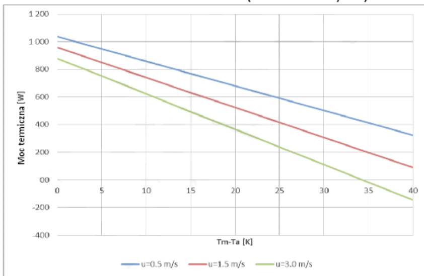
WYDAJNOŚĆ KOLEKTORA (dla G=1000\text{W}/\text{m}^2 )
