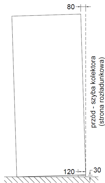
2.1 Pozycja rozładunkowa
